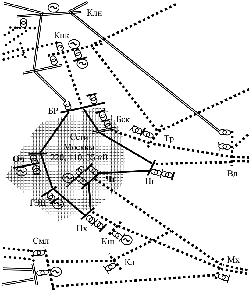
Рис.4.6. Схема московского кольца 500 кВ к аварии 25.05.2005
