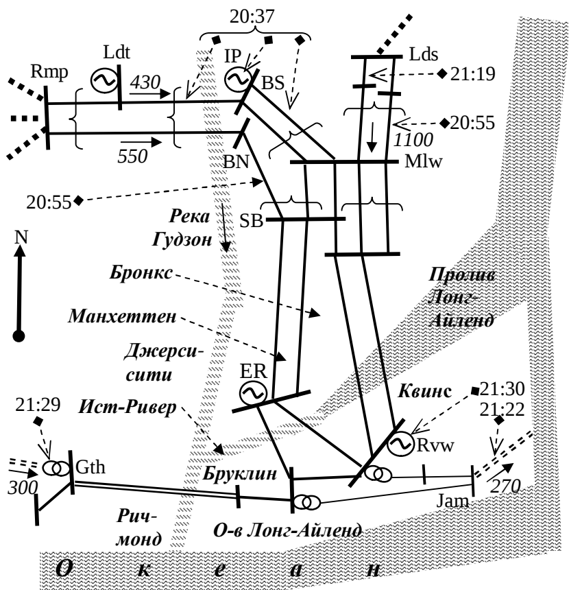
Рис.4.3. Упрощенная схема электроснабжения Нью-Йорка к аварии 13.07.1977
